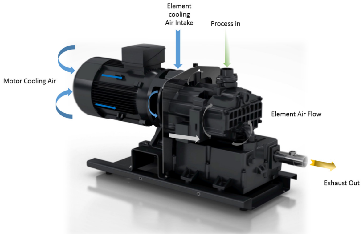
Охлаждение насоса
