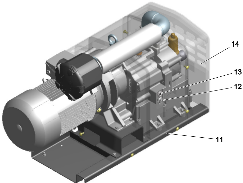
Нагнетательные безмасляные кулачковые насосы DZS 150P, DZS 300P, вид спереди
