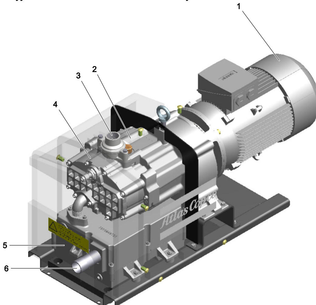
Вакуумные безмасляные кулачковые насосы DZS 065V, DZS 150V, DZS 300V, вид сзади
