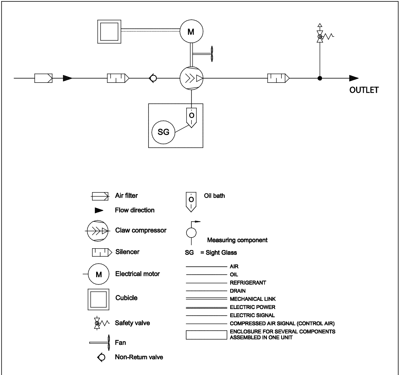
Схема потока - нагнетательные безмасляные кулачковые насосы DZS 150P, DZS 300P
