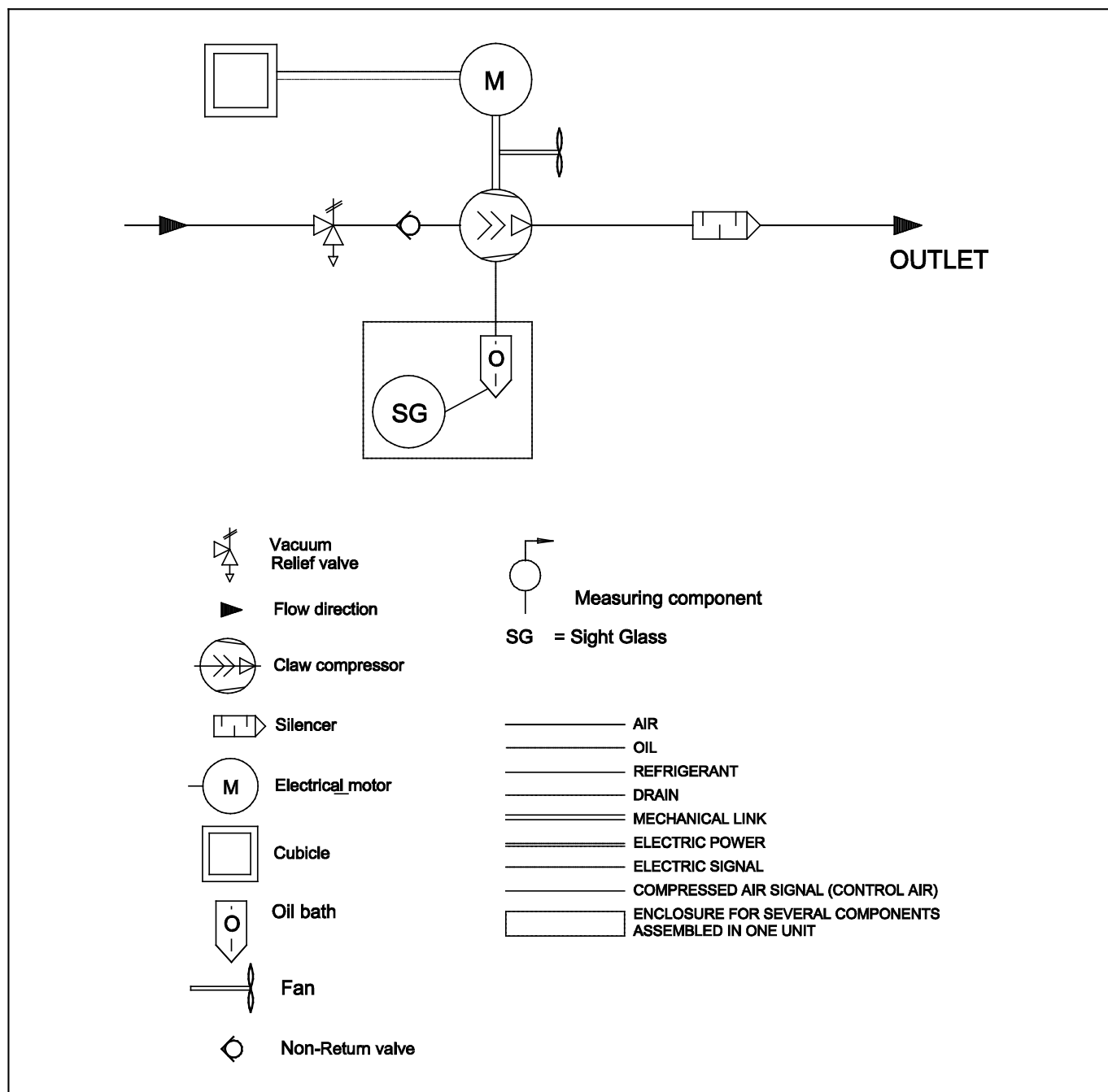
Схема потока - вакуумные безмасляные кулачковые насосы DZS 065V, DZS 150V, DZS 300V
