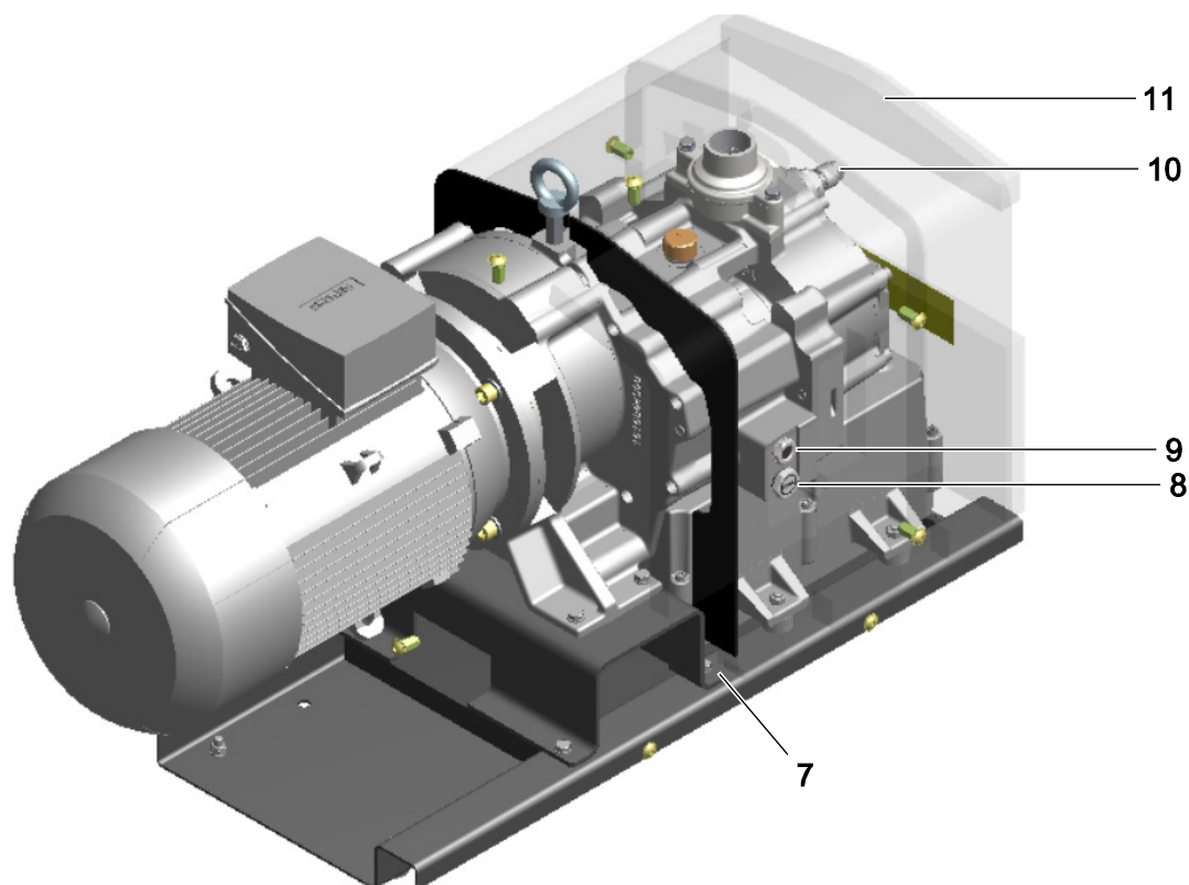
Вакуумные безмасляные кулачковые насосы DZS 065V, DZS 150V, DZS 300V, вид спереди
