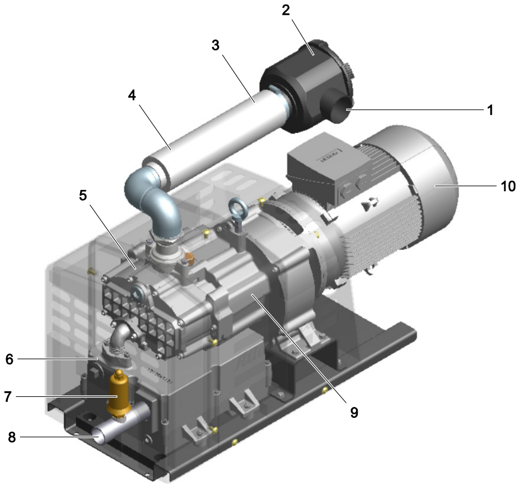
Нагнетательные безмасляные кулачковые насосы DZS 150P, DZS 300P, вид сзади
